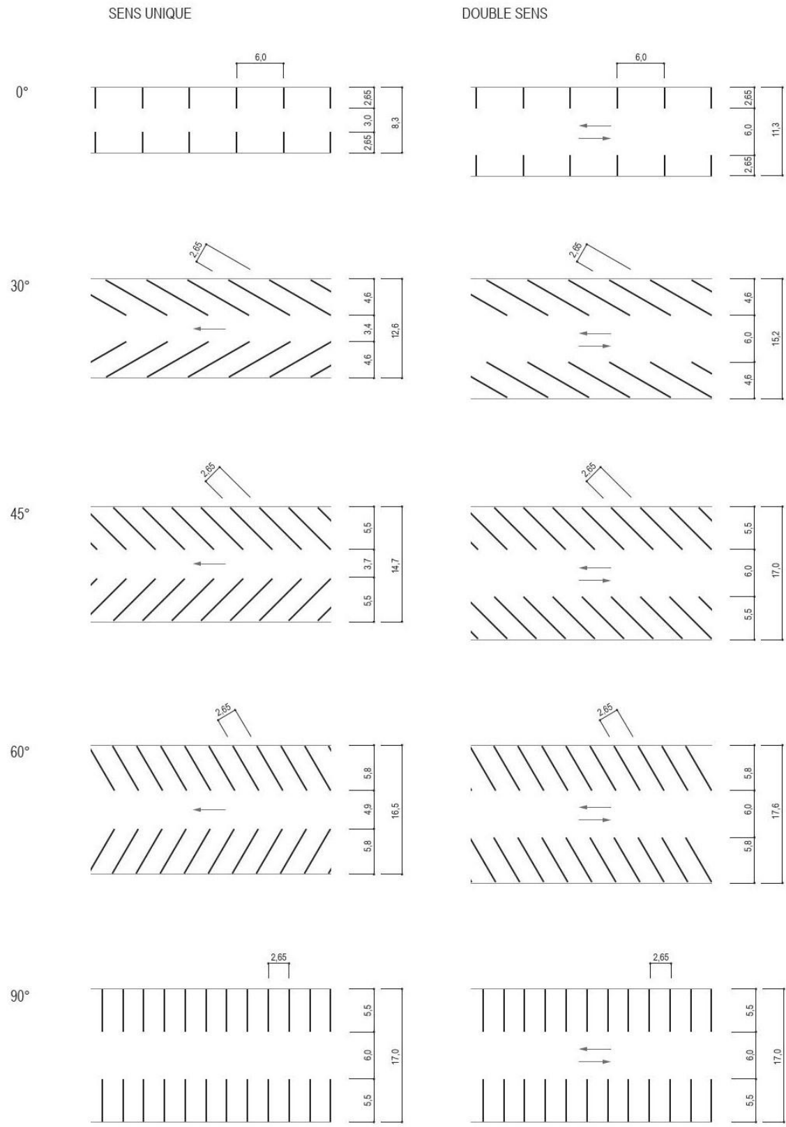
Figure 6.1 : Dimensions d’une aire de stationnement
