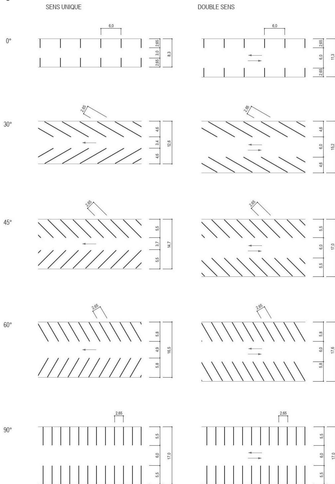
Figure 7.1 : Dimensions d'une aire de stationnement
