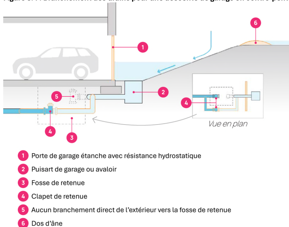
Figure 3.4 : Branchement des drains pour une descente de garage en contre-pente
