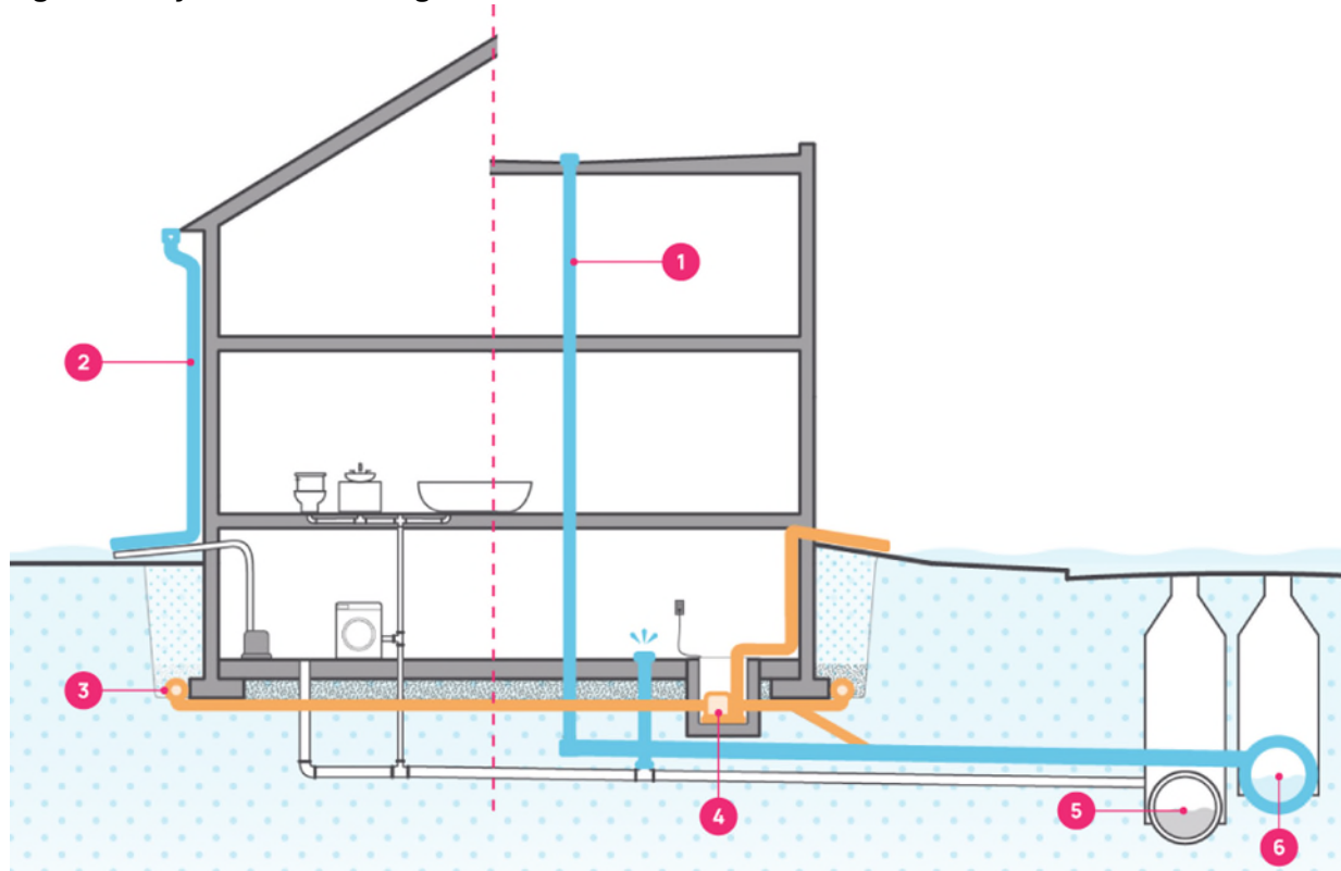
Figure 3.1 : Systèmes de drainage des eaux extérieures
