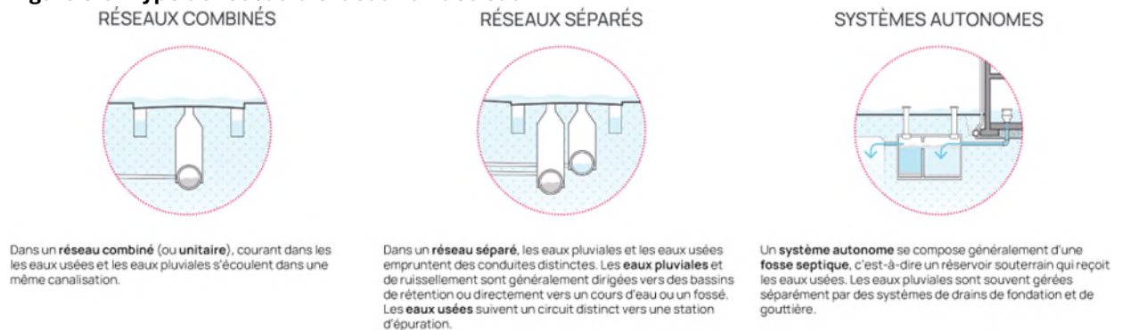
Figure 3.5 : Type de réseau d'évacuation des eaux
