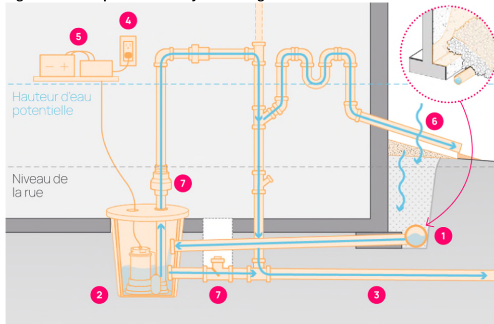
Figure 3.3 : Composition d'un système de gestion des eaux souterraines
