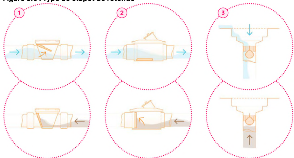
Figure 3.6 : Type de clapet de retenue
