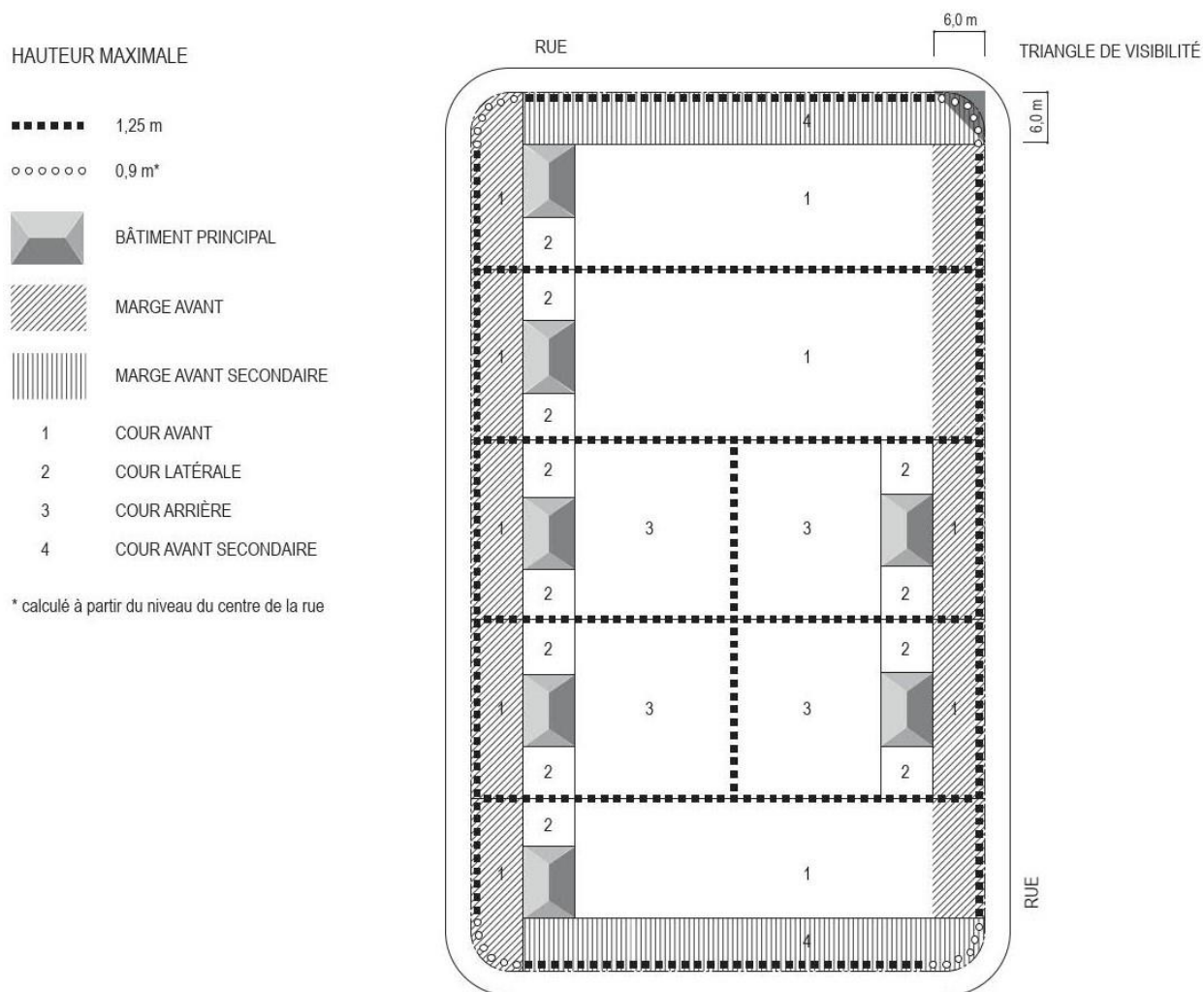
Figure 6.6 : Hauteur maximale autorisée pour un muret (terrain intérieur, terrain d'angle transversal et terrain transversal)
