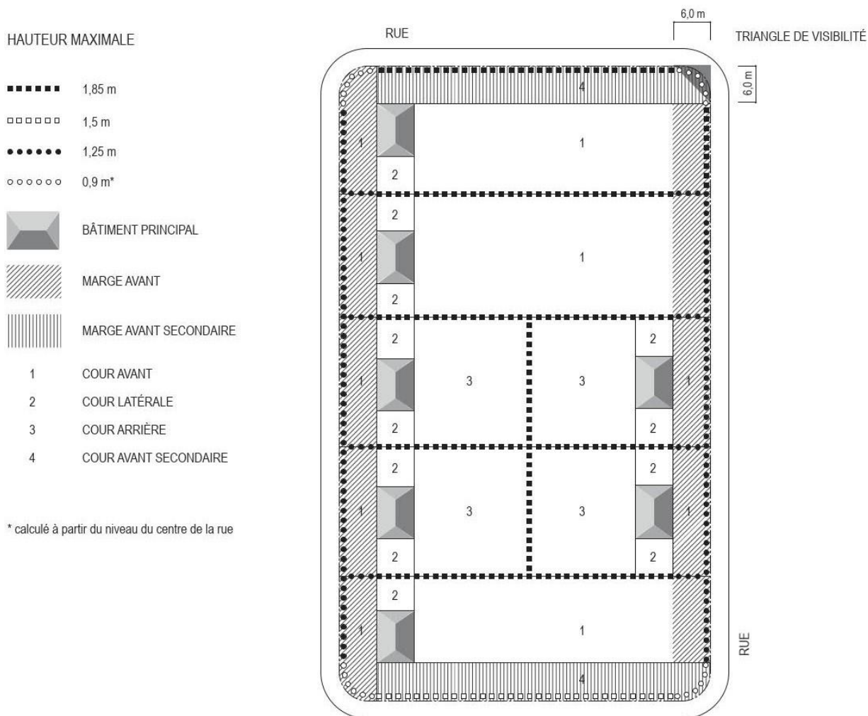
Figure 7.4 : Hauteur maximale autorisée pour une clôture (terrain intérieur, terrain d'angle transversal et terrain transversal)
