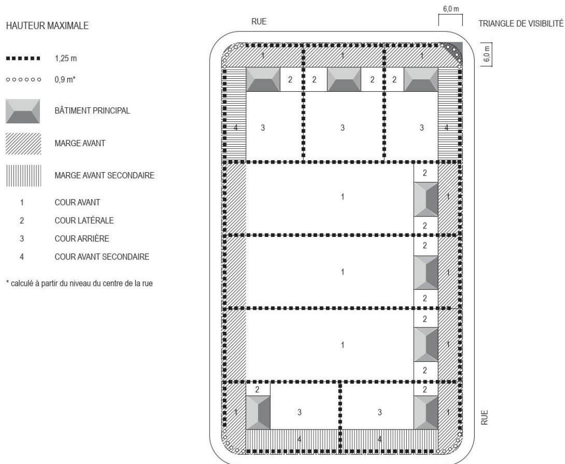
Figure 7.5 : Hauteur maximale autorisée pour un muret (terrain intérieur, terrain d'angle et terrain transversal)
