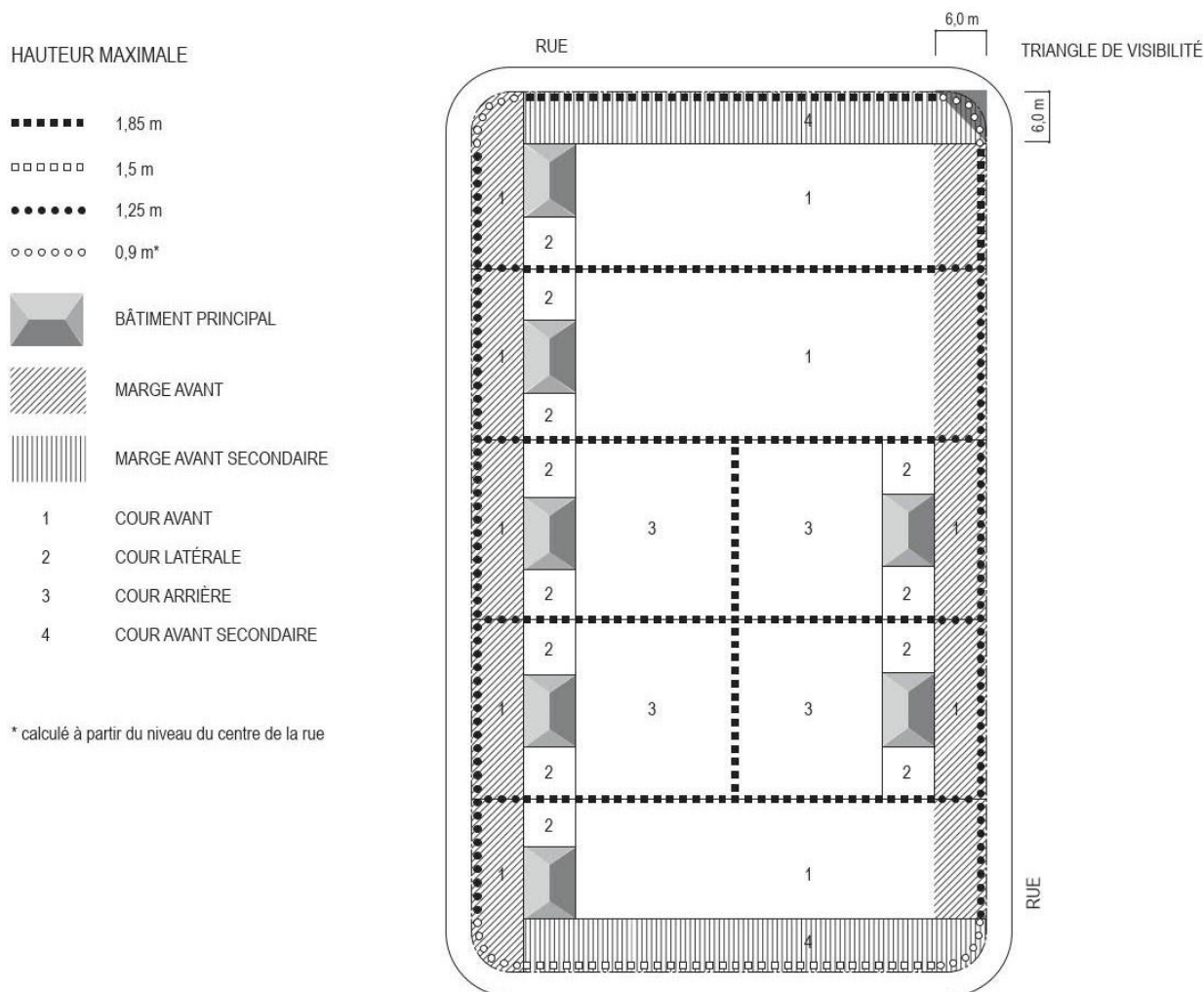
Figure 6.4 : Hauteur maximale autorisée pour une clôture (terrain intérieur, terrain d'angle transversal et terrain transversal)
