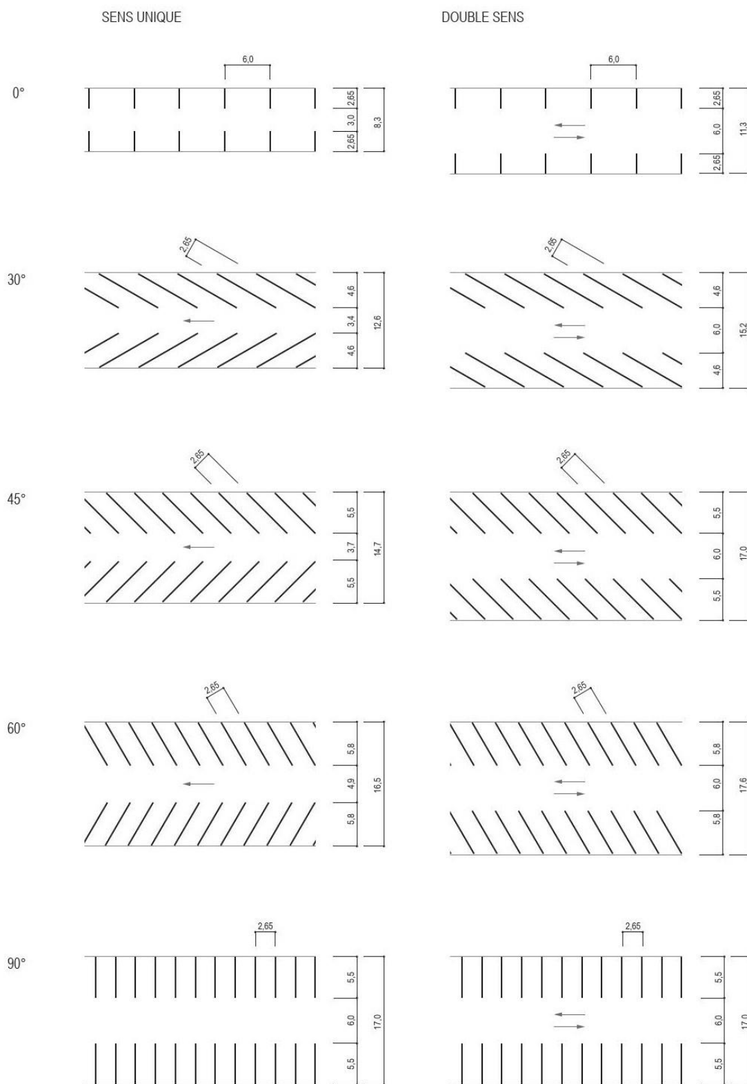
Figure 6.1 : Dimensions d'une aire de stationnement
