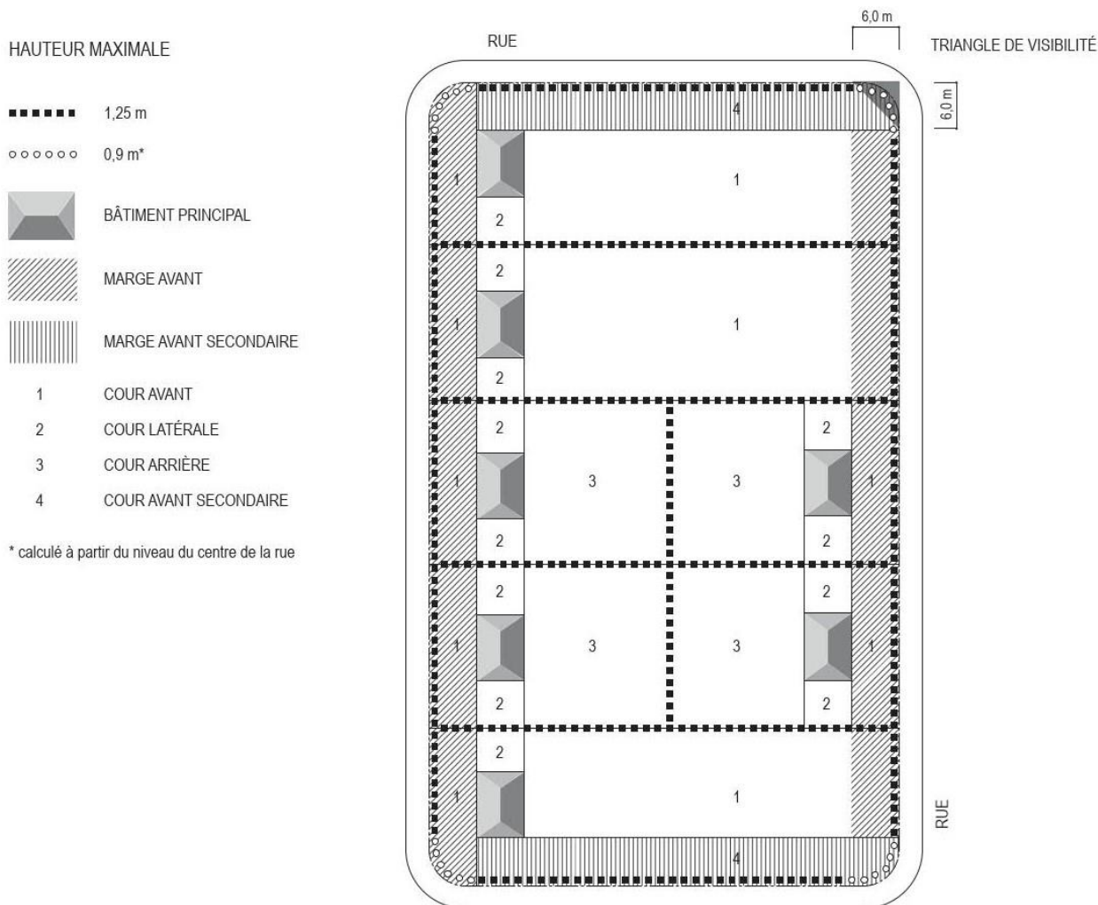
Figure 7.6 : Hauteur maximale autorisée pour un muret (terrain intérieur, terrain d'angle transversal et terrain transversal)
