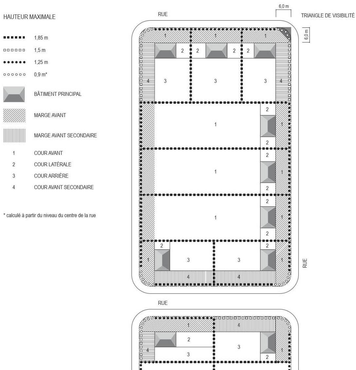
Figure 6.3 : Hauteur maximale autorisée pour une clôture (terrain intérieur, terrain d'angle et terrain transversal)
