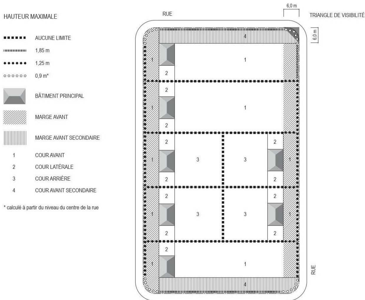
Figure 7.8 : Hauteur maximale autorisée pour une haie (terrain intérieur, terrain d'angle transversal et terrain transversal)
