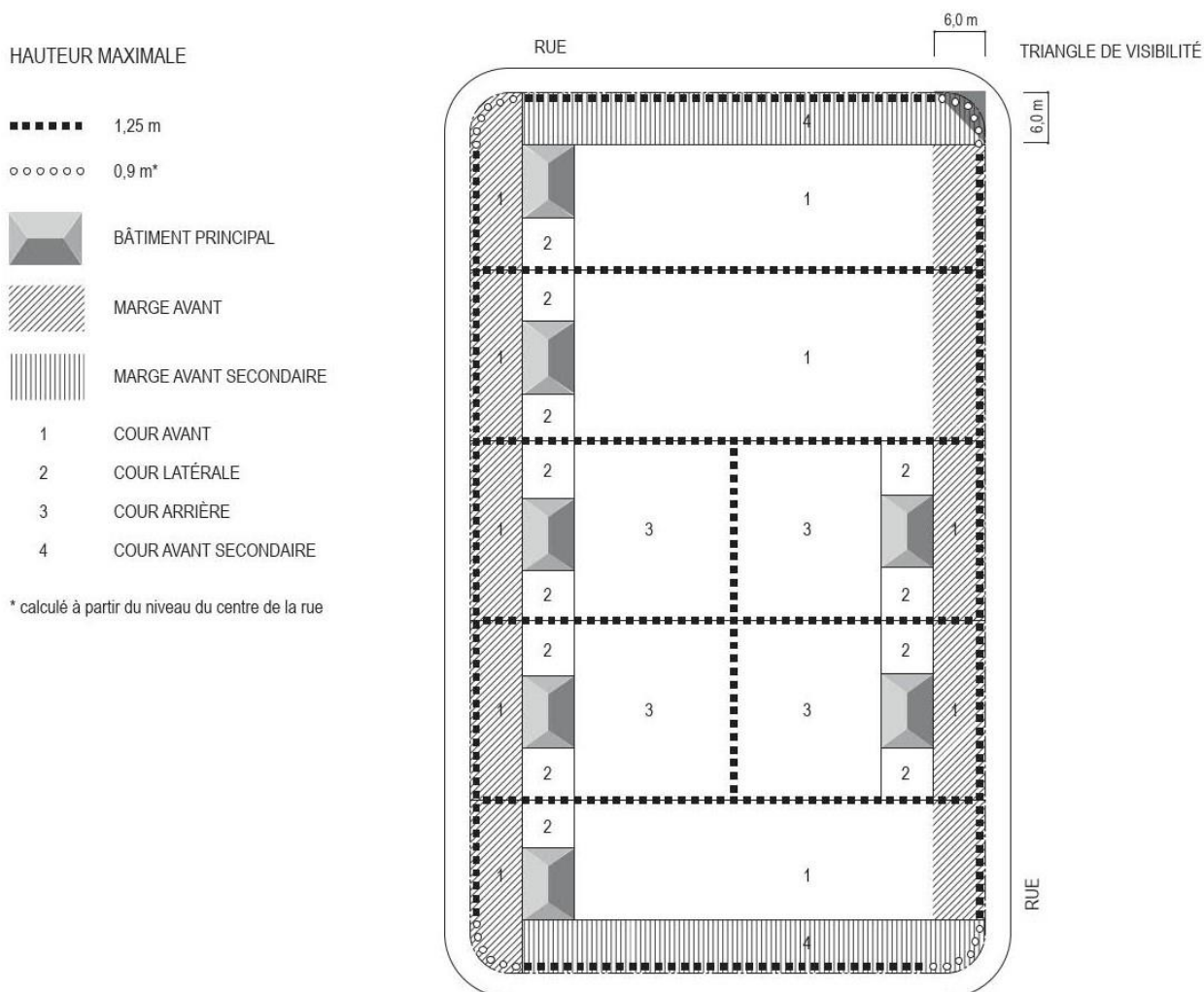
Figure 6.8 : Hauteur maximale autorisée pour une haie (terrain intérieur, terrain d'angle transversal et terrain transversal)
