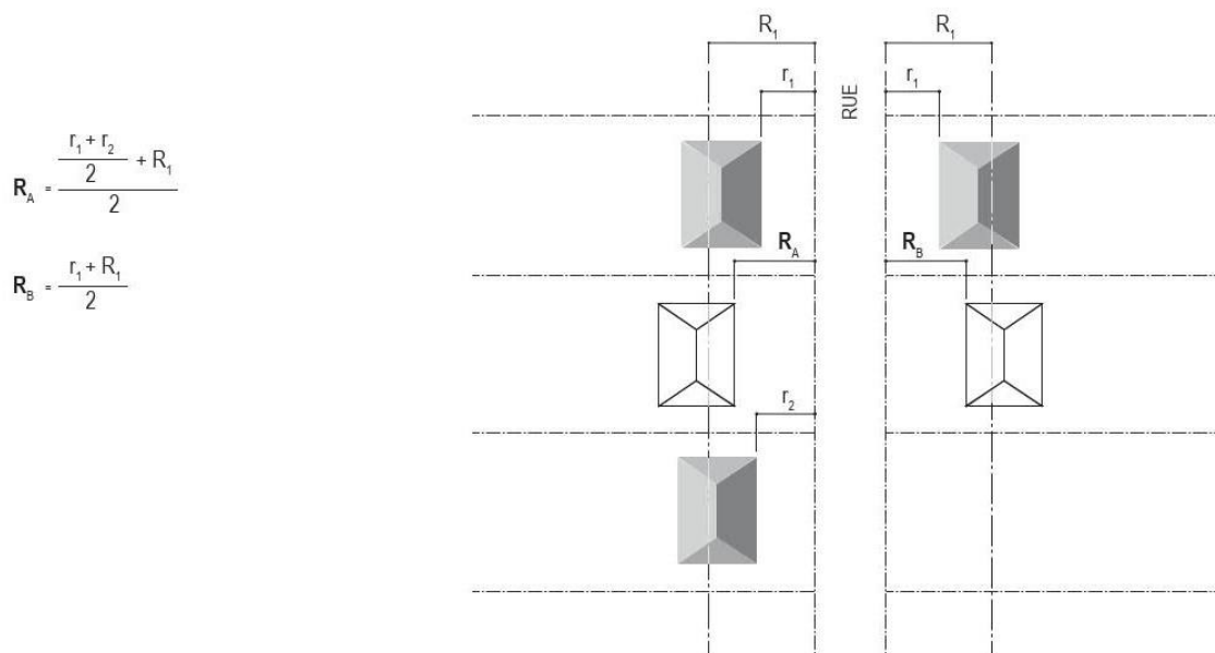
Figure 5.3 : Marge avant minimale réduite
