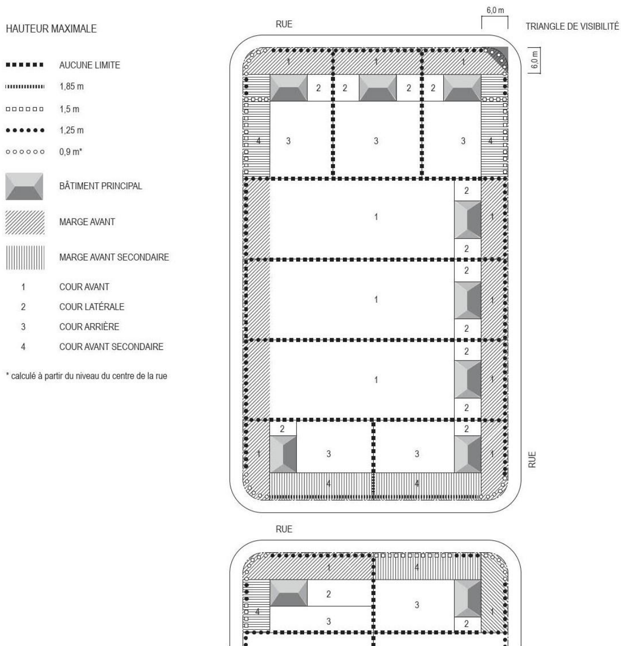
Figure 6.7 : Hauteur maximale autorisée pour une haie (terrain intérieur, terrain d'angle et terrain transversal)
