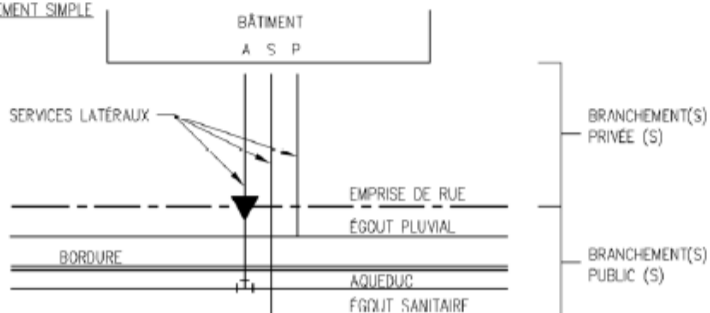
BRANCHEMENT SIMPLE
